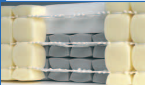
16 cm – dreischichtig
