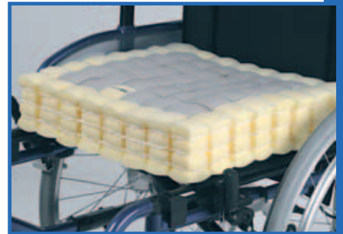
10 cm – zweischichtig
